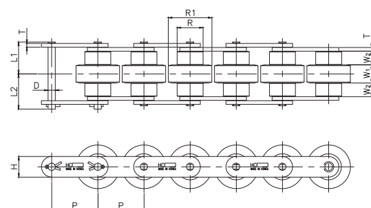
CR(VR)-NC : 커버 없음
