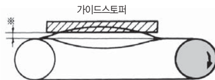
※ 체인과 접촉면과의 틈새 2~4mm
