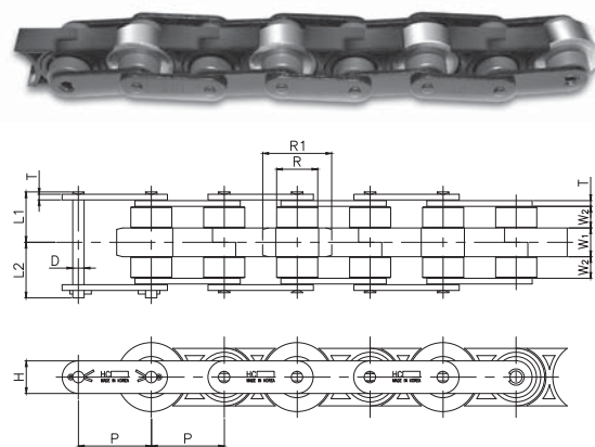
CR(VR) : 센터블록 (2L/대롤러용)
