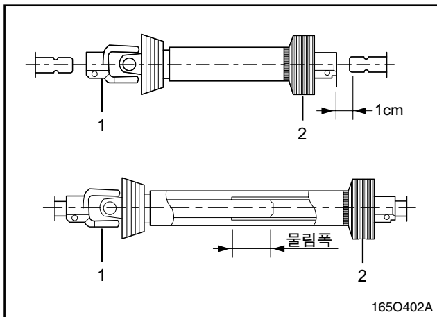
(1) 트랙터 PTO축
